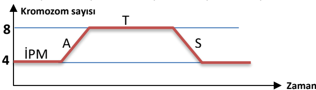
2n=4 Kromozumlu bir hücrenin Mitoz bölünmesindeki kromozom sayısı değişimi grafiği
