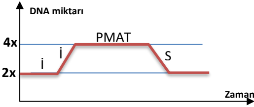
Mitoz hücre bölünmesindeki DNA miktarı değişimi grafiği
